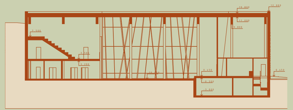
řez B
